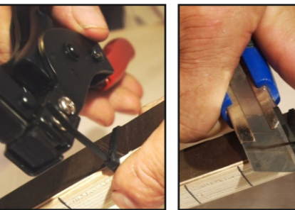
Plaats de de bandjes op de lijntjes op de hals. De knoop van elk bandje zit op de hoek van de hals, bovenaan aan de voorkant. Trek zéér hard aan met een tangske zodat het bandje zeer strak rond de hals vast zit.
