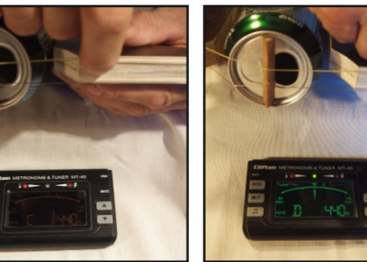
Span de snaren op door aan de knoppen van de stemmechaniek te draaien. Stem de snaren naargelang de dikte bv. in D en G. De dunste snaar (de onderste) klinkt even hoog als de dikste op de 7de fret gedrukt.
