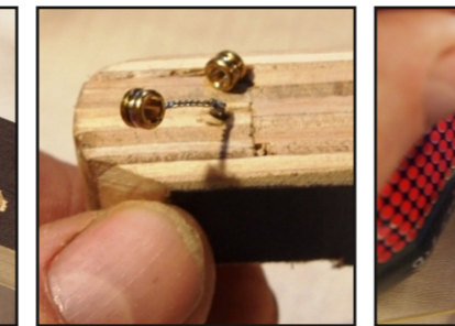
Steek de snaren langs de onderkant in door de gaatjes in de hals, dikste snaar (dunne) in de onderste stemmechaniek.
