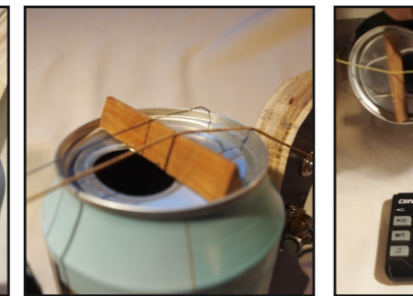
Verwijder de klips van het blik. Plaats driehoekige houten brug zoals op de foto in het midden van het blikje. Plaats de snaren in de inkepingen en steek de uiteinden in de gaatjes van de stemmechanieken.
