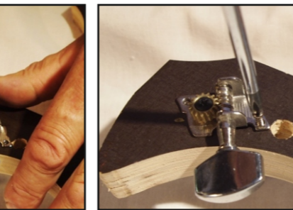
Steek de stemmechaniek langs de andere zijde in het gatje. Het tandwieletje naar boven gericht. Schroef de schroefjes door de gaatjes in de voorgeprikte putjes.
