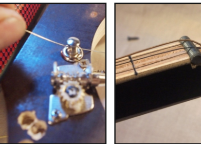
Aan de andere kant in de stemmechaniek. De onderste snaar (dunne) in de onderste stemmechaniek.
